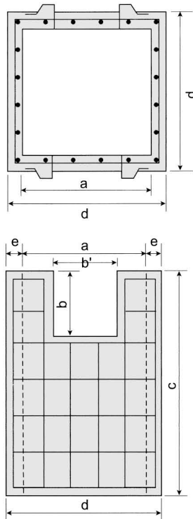
分水柵本体
