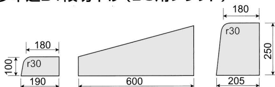
(B-1) 片面歩車道B1段切下げ(BC用フラット)
