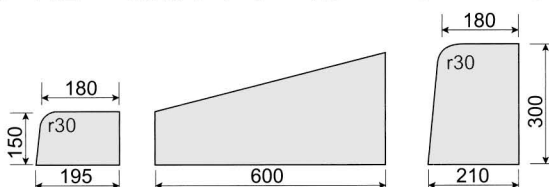
(C-1) 片面歩車道C1段切下げ(BC用フラットH150)
