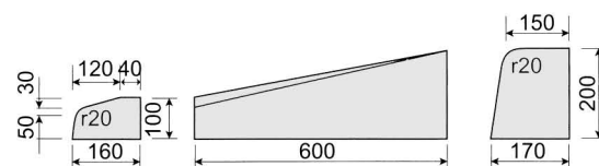
(A-2) 片面歩車道A1段切下げ(A用バイコロジー)
