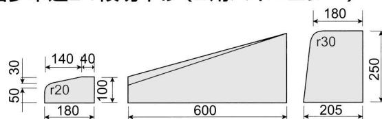
(B-2) 片面歩車道B1段切下げ(B用バイコロジー)
