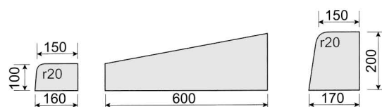
(A-1) 片面歩車道A1段切下げ(A用フラット)
