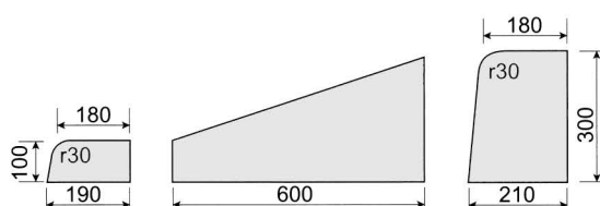
(C-3) 片面歩車道C1段切下げ(BC用フラット)
