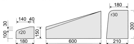
(C-2) 片面歩車道C1段切下げ(B用バイコロジーH150)
