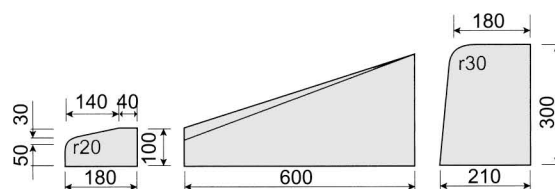
(C-4) 片面歩車道C1段切下げ(B用バイコロジー)
