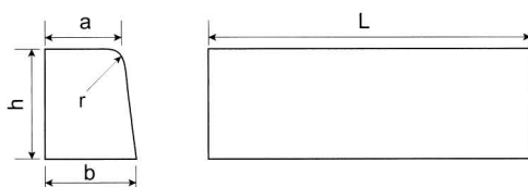
片面歩車道境界ブロック (水抜)
