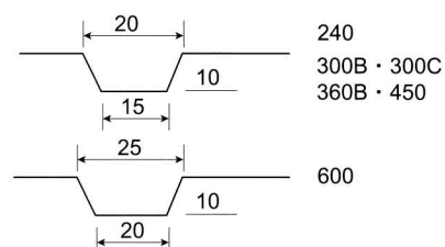
仕切版詳細
