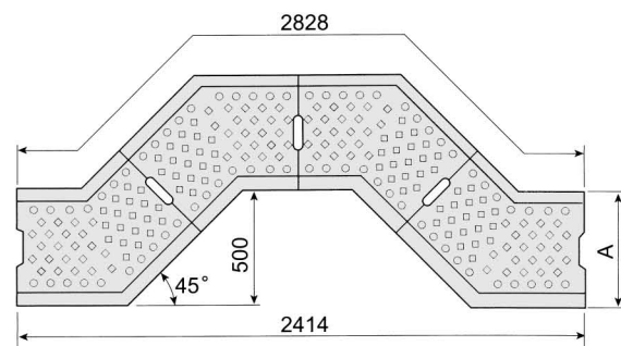
布設平面図
