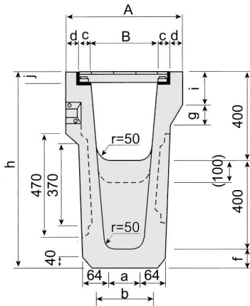
PU3・4G型用溜槽
