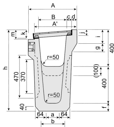
PU6 G型用溜槽
